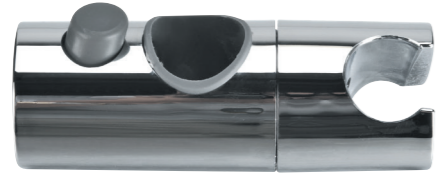
SB3000 Diameter: φ 18mm φ 20.5mm φ 22mm φ 23mm φ 24mm φ 25mm
