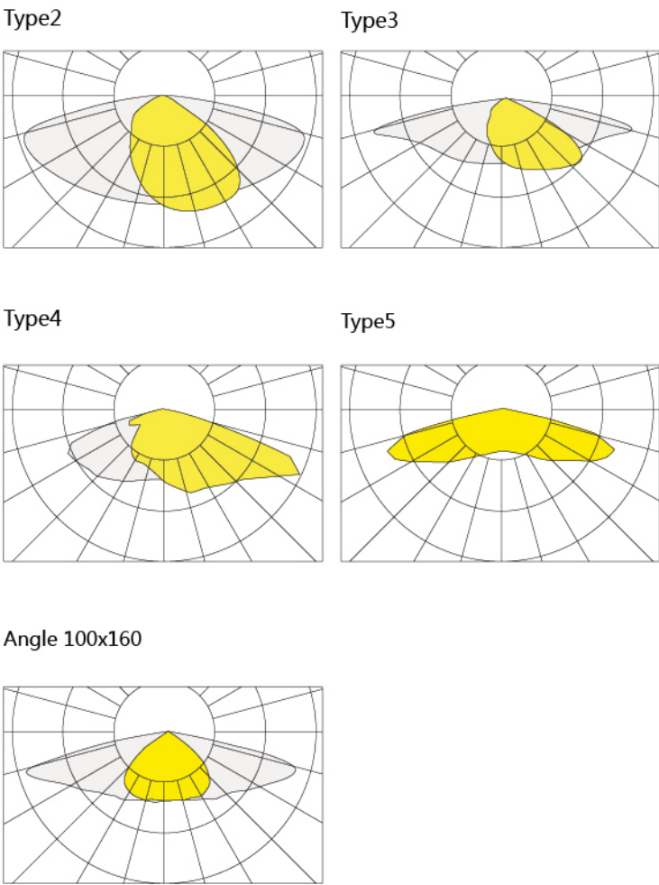
配光曲线 Polar Diagram
