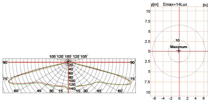
配光曲线 Polar Diagram
