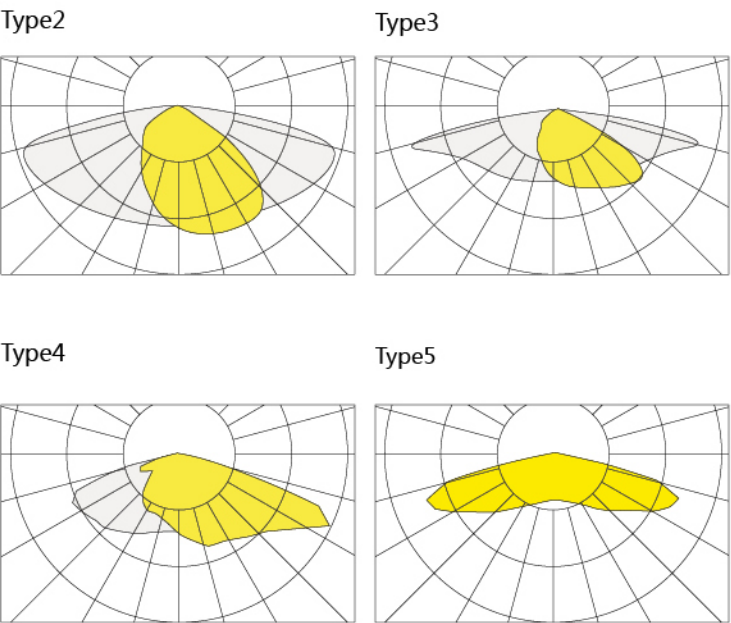
配光曲线 Polar Diagram
