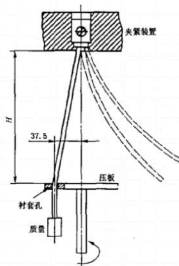
图1 弯曲试验的试验设备 (见 8.2.4.3 和表 5)
