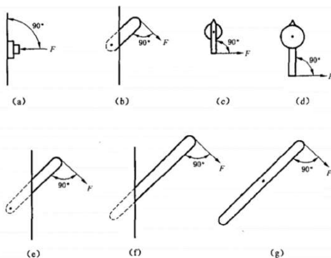
图 16 操动器试验力 (8.2.5.2.1 和表 17)
