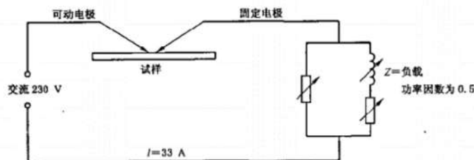
图 M.2 电弧引燃试验电路图
