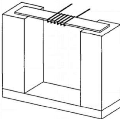
图 M.1 电热丝引燃试验装置
