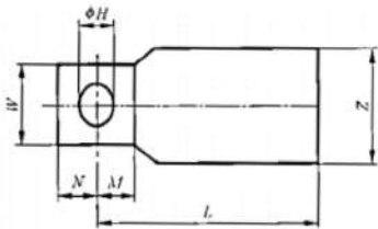
图 P.1 尺寸
