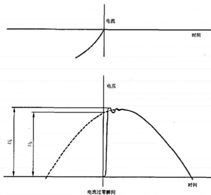
图 7 在理想条件下,首先熄弧触头两端的恢复电压的简单示意图 (见 8.3.3.5.2 e))
