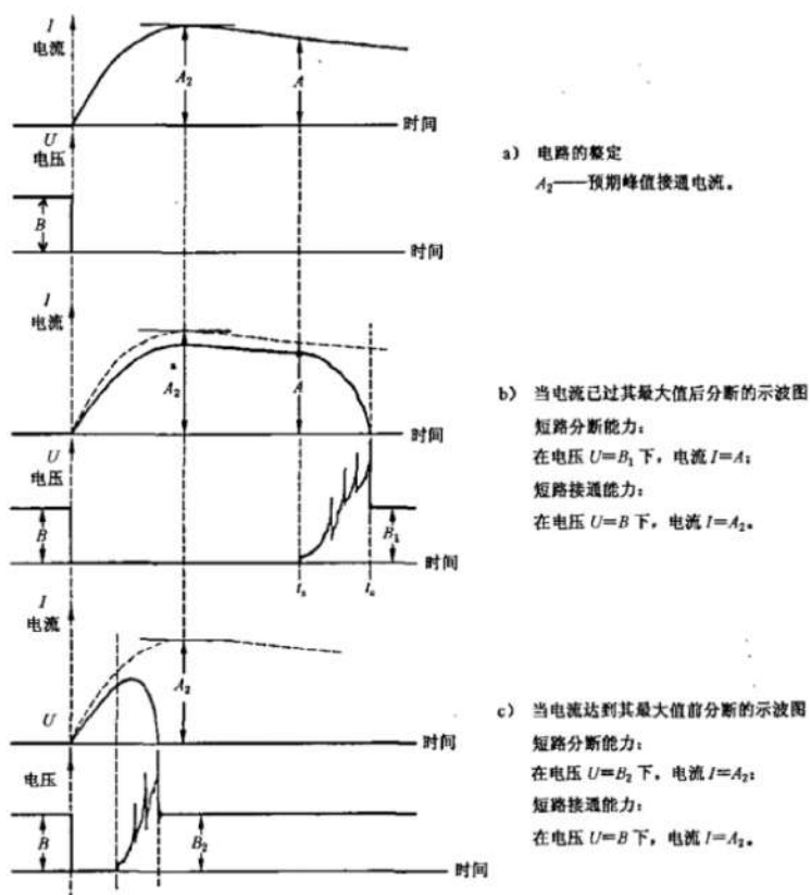
图 14 验证直流短路接通和分断能力 (见 8.3.4.1.8)
