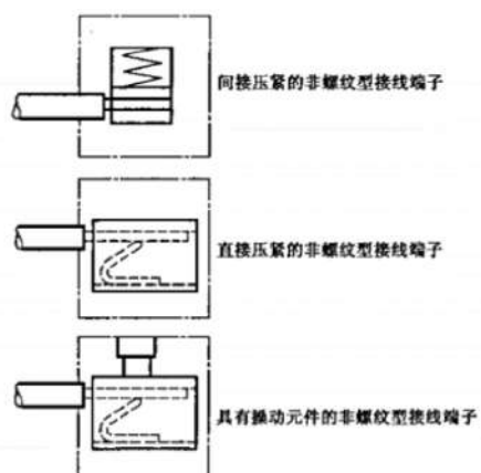
图 D.7 非螺纹型接线端子
