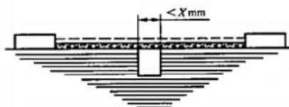
图 G.2 触头支持用固定的和移动的绝缘件间的爬电距离
