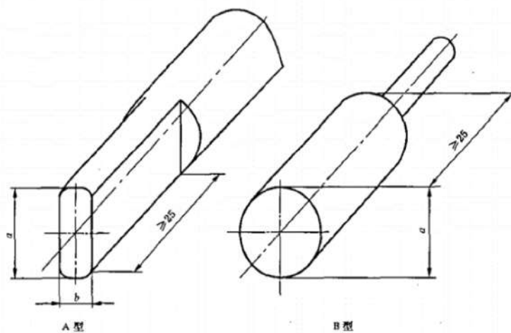
图2 A型和B型模拟量规 (见 8.2.4.5.2 和表 7)
