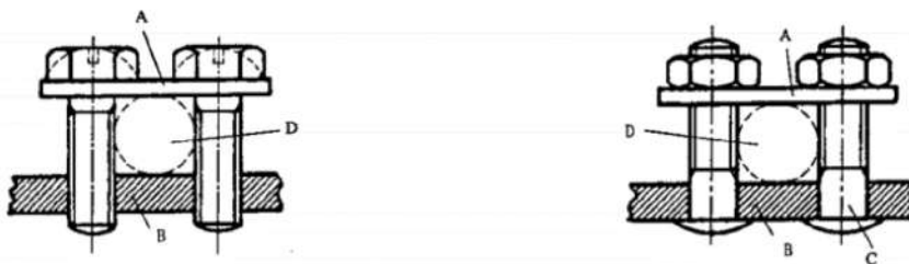
图 D.3 螺栓型接线端子
