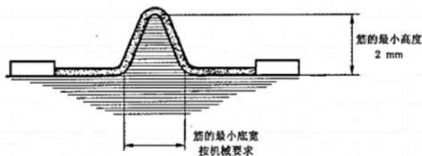
图 G.1 筋的测量
