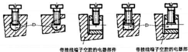
无压板的接线端子
