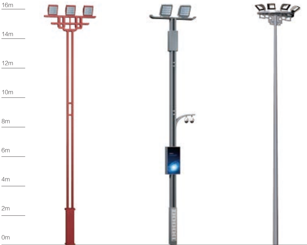
型号: LDZG-16401 型 型号: LDZG-16402 型 型号: LDZG-16403 型
