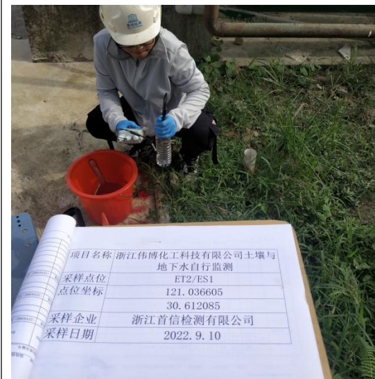
照片3： 洗井监测
