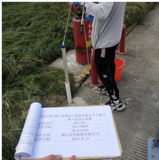
照片11： 地下水采样
