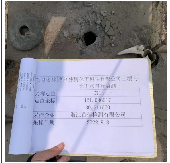
照片3： 完成钻 孔
