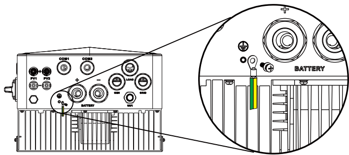
Conexão de aterramento (fios de cobre)
