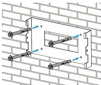
Instalação da placa suspensa do inversor
