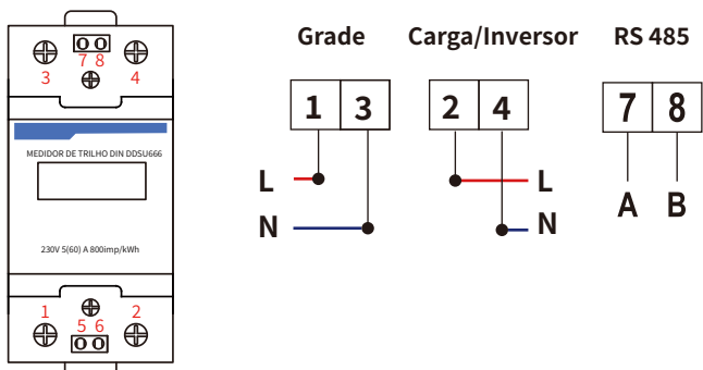
CHINT DDSU666
