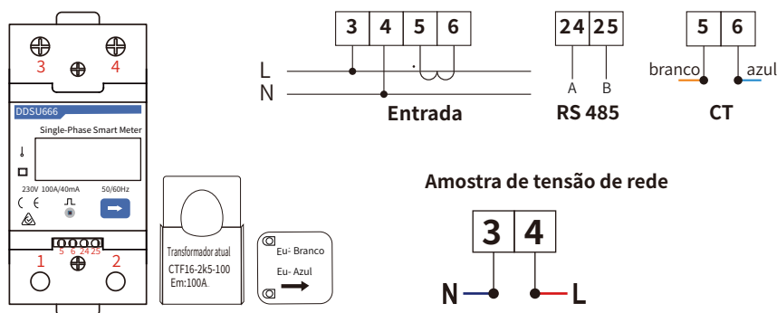
Figura 7.9 Medidor CHINT
