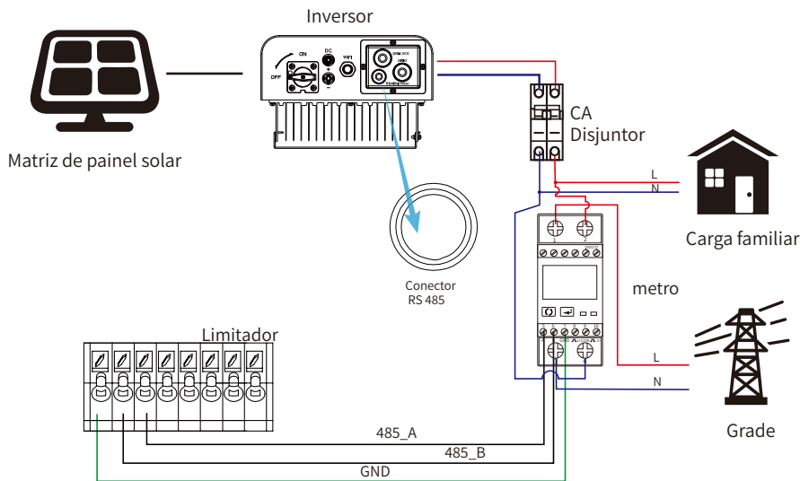
Figura 7.2 Diagrama de conexão do medidor EASTRON
