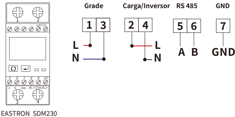
Figura 7.11 Medidor EASTRON
