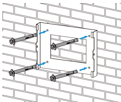
Instalação da placa suspensa do inversor
