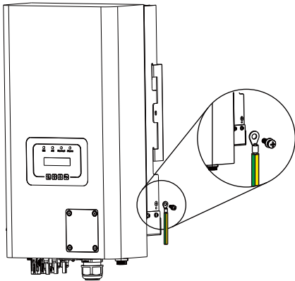
Imagen 5.8 La instalación del cable de tierra de la carcasa
