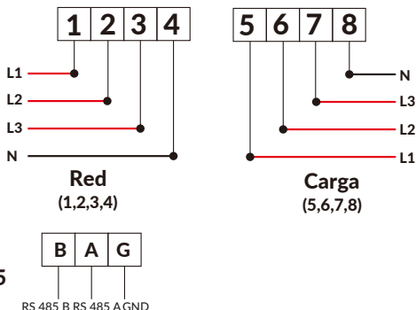
Imagen 7.1 Medidor Eastron
