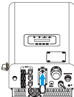
Imagen 5.10 Diagrama de instalación del registrador de datos
