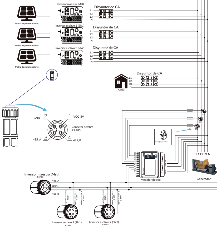
Imagen 7.25 Diagrama de conexión (electricidad trifásica)
