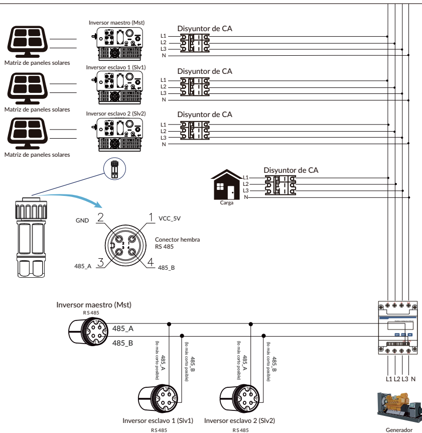
Imagen 7.29 Diagrama de conexión CHINT (tabla de paso)
