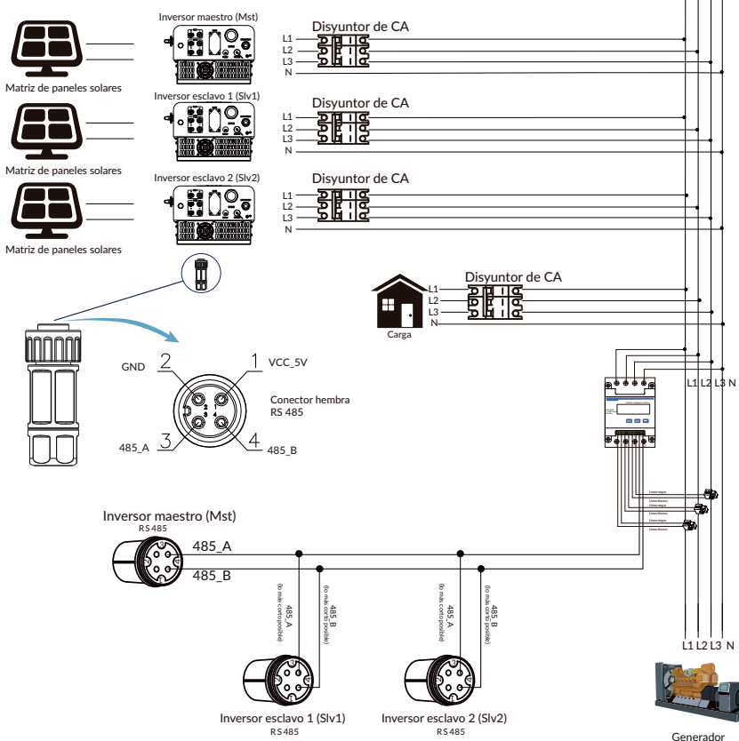
Imagen 7.33 Diagrama de conexión CHINT (tabla de paso)
