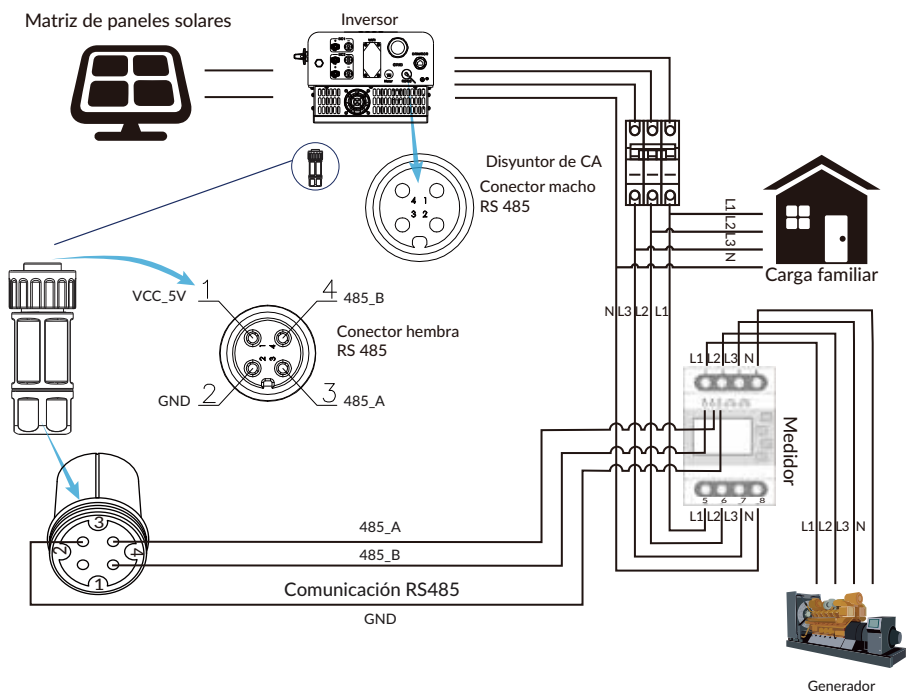
Imagen 7.4 Diagrama de conexión del medidor Eastron
