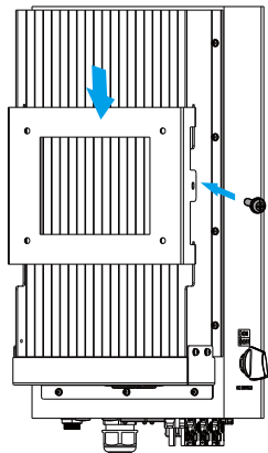
Imagen 4.6 Instalación del inversor
