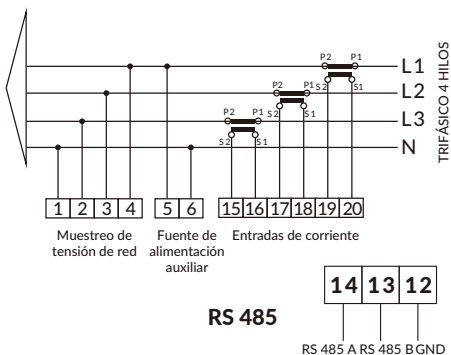
Imagen 7.7 Medidor Eastron
