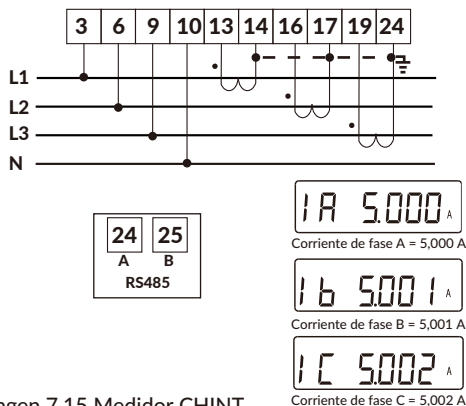
Imagen 7.15 Medidor CHINT
