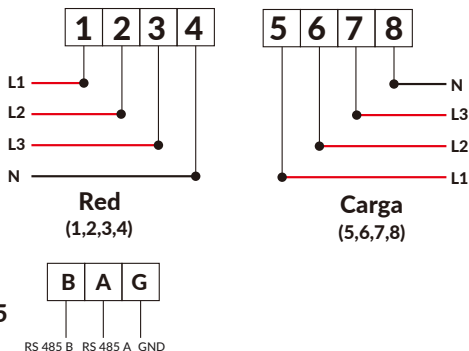
Imagen 7.18 Medidor Eastron
