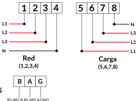
Imagen 7.3 Medidor Eastron
