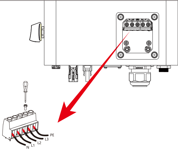
Imagen 5.7 Conexión de entrada de CA
