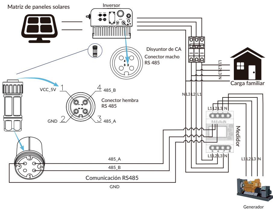
Imagen 7.4 Diagrama de conexión del medidor Easton
