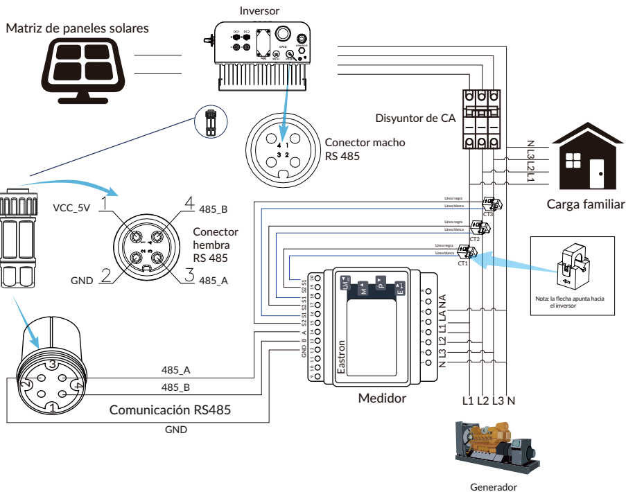
Imagen 7.8 Diagrama de conexión del medidor Eastron
