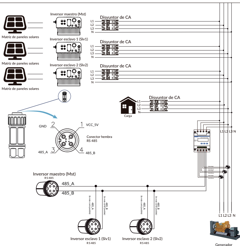
Imagen 7.33 Diagrama de conexión CHINT (tabla de paso)
