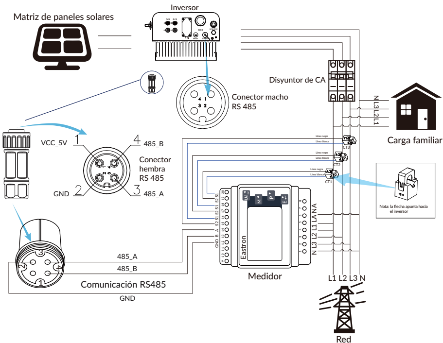
Imagen 7.6 Diagrama de conexión del medidor Eastron
