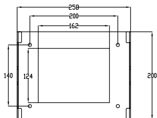
Imagen 4.5 Instalación de la placa de suspensión del inversor
