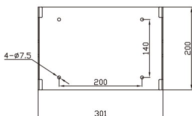
Image 4.5 Installation de la plaque de suspension de l'onduleur
