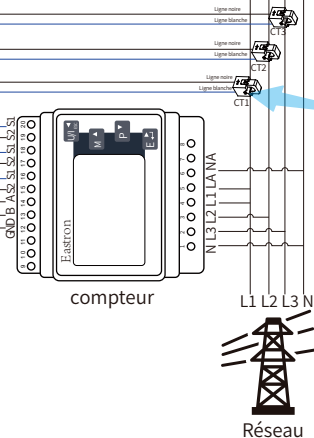
Image 7.6 Schéma de connexion du compteur Eastron
