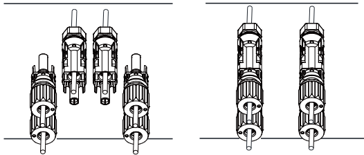
Fig. 5.6 Conexión de la entrada de CC
