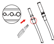
图5.4 将压接端子压接到电线上
