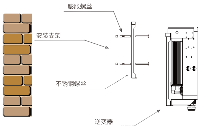
图4.5 逆变器的安装
