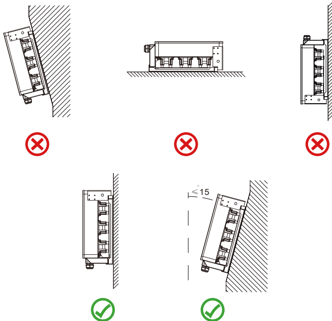
图4.2 安装角度
