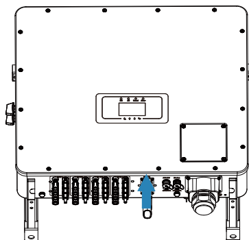
图5.14 数据采集器的安装
