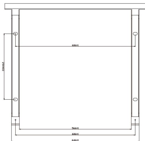
图 4.4 支架尺寸
