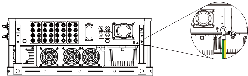
图5.12 外壳接地线的安装
