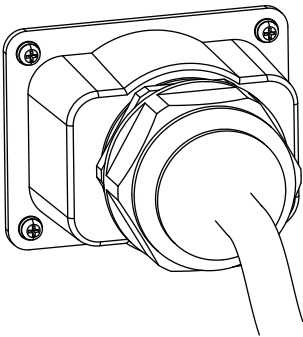
图5.11 拧紧AC接线盒
