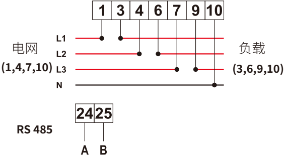
图7.5 正泰电表
