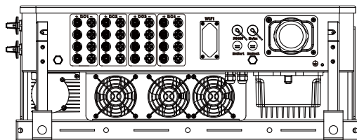
图1.2 底视图
