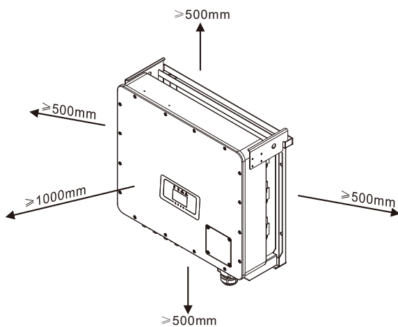
图4.3 安装间隙
