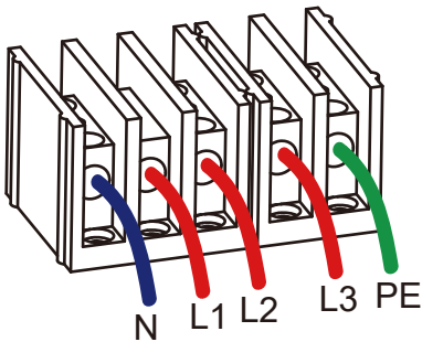
图5.9 AC电缆连接端子
