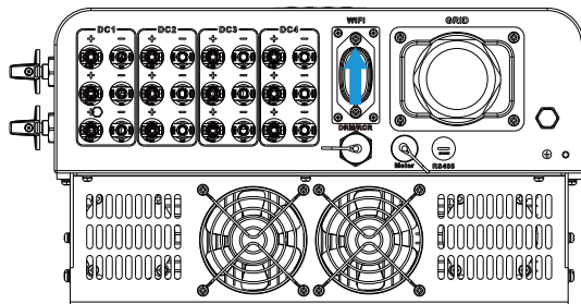
Imagen 5.10 Diagrama de instalación del registrador de datos
