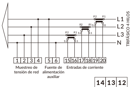
Imagen 7.5 Medidor Eastron
