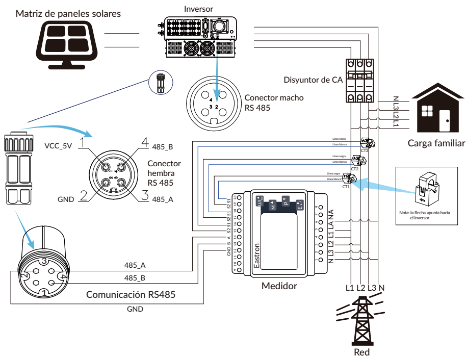
Imagen 7.6 Diagrama de conexión del medidor Eastron
