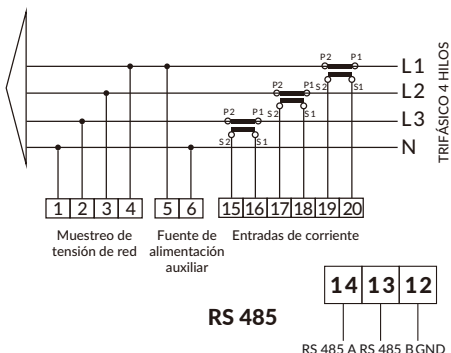
Imagen 7.7 Medidor Eastron
