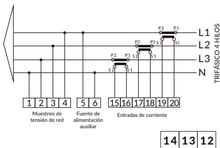
Imagen 7.24 Medidor Eastron
