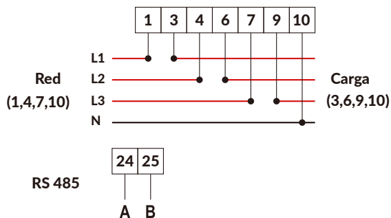
Imagen 7.28 Medidor CHINT
