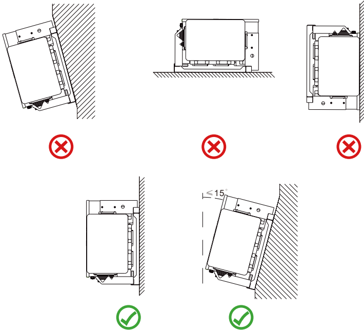
图4.2 安装角度
