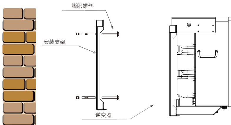
图4.5 逆变器的安装
