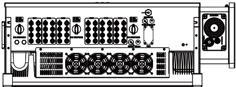
图1.2 底视图
