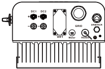
图1.2 底视图
