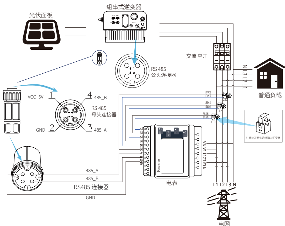
图6.4 东鸿三相电表连接
