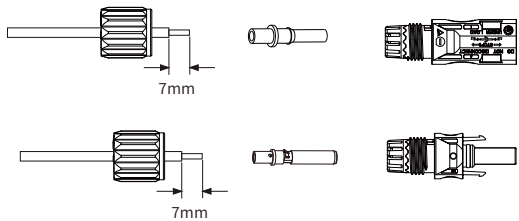
图5.3 拆卸连接器螺帽
