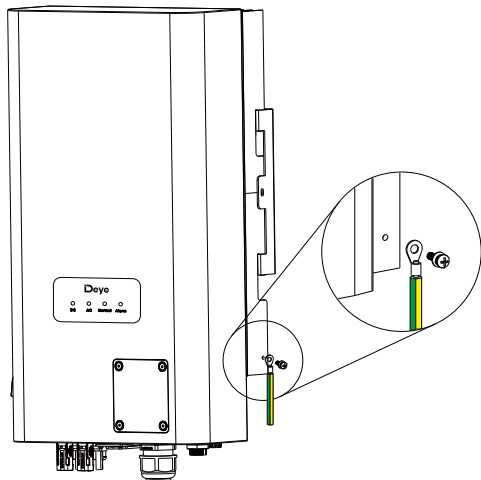
图5.11 外壳接地线的安装
