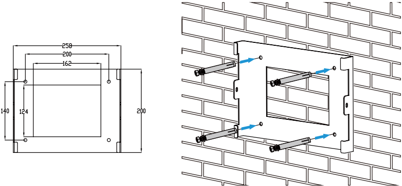
图4.5 逆变器支架的安装
