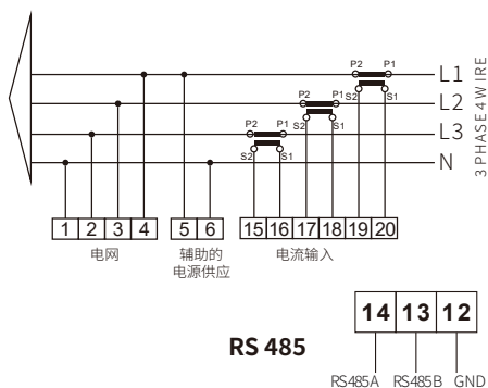
图6.3 东鸿三相电表
