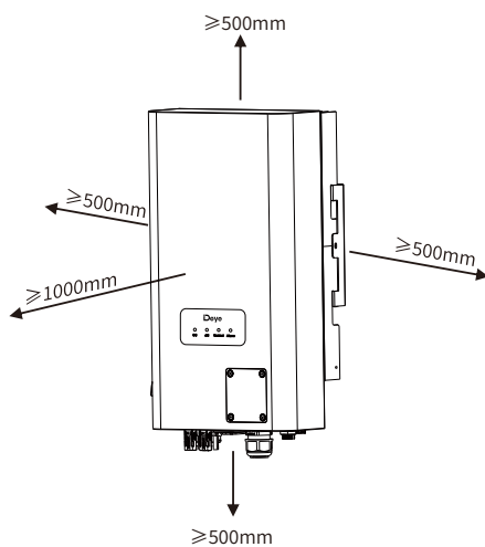
图4.3 安装间隙
