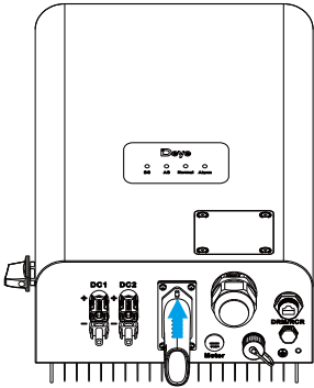
图5.13 数据记录仪安装图示
