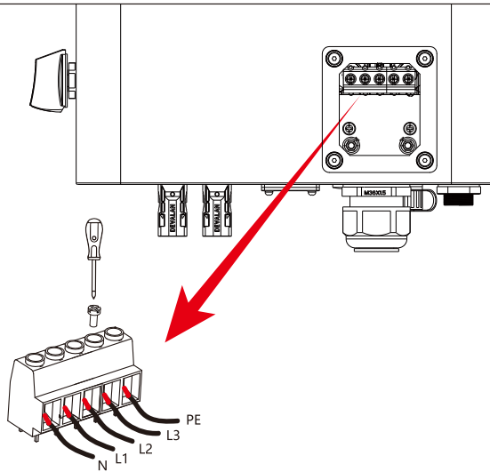
Abb. 5.7 AC-Eingangsanschluss
