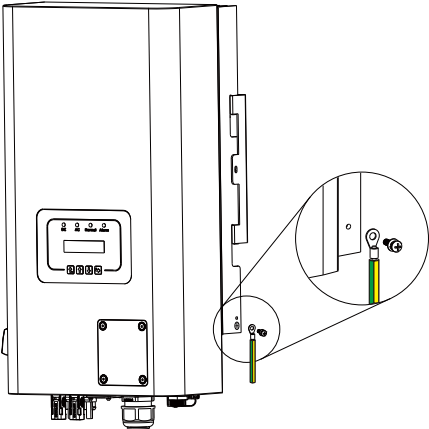
Abb. 5.8 Installation des Mantelerdungsdrahtes
