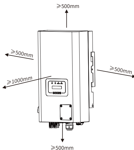
Abb. 4.3 Einbaulücke
