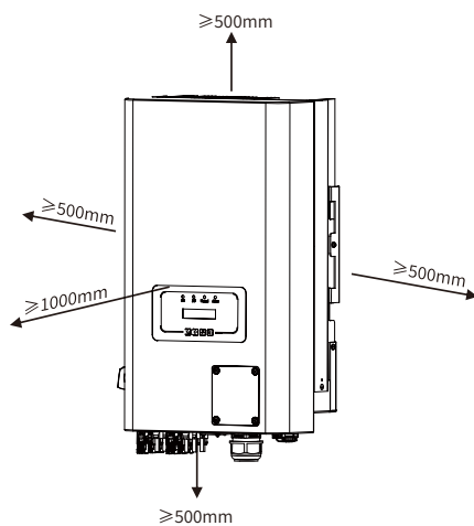
Abb. 4.3 Einbaulücke
