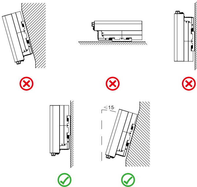
Abb. 4.2 Einbauwinkel
