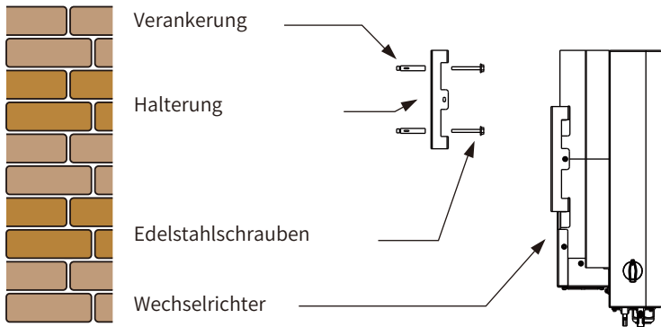
Abb. 4.4 Installation des Wechselrichters
