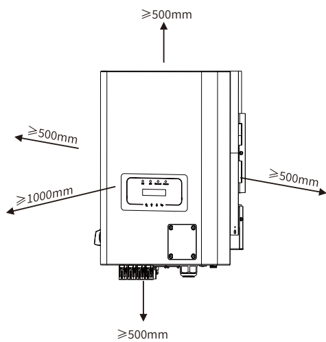
Abb. 4.3 Einbaulücke
