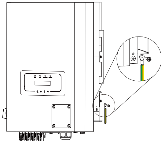
Abb. 5.11 Installation des Mantelerdungsdrahtes
