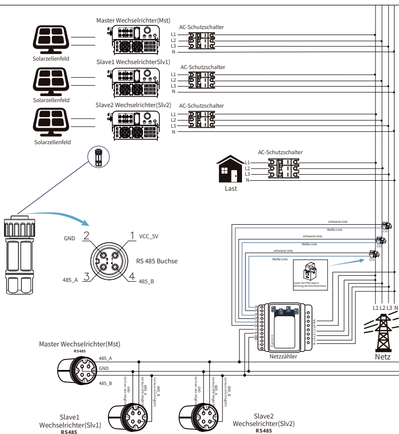
Abb. 7.23 Anschlussplan (Dreiphasenstrom)
