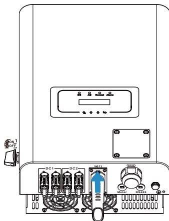
Abb. 5.13 Installationsschema des Datenloggers
