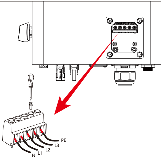
Abb. 5.7 AC-Eingangsanschluss
