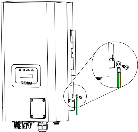
Abb. 5.8 Installation des Mantelerdungsdrahtes
