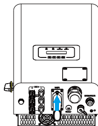
Abb. 5.14 Installationsschema des Datenloggers
