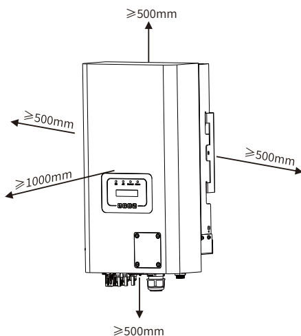
Abb. 4.3 Einbaulücke
