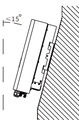
Abb. 4.2 Einbauwinkel
