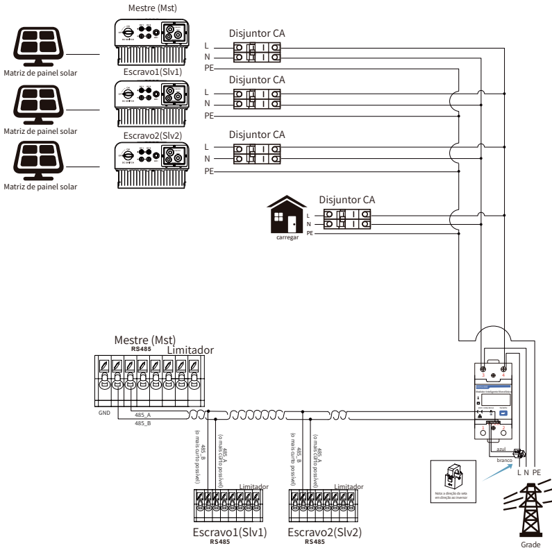
Pic 7.17 Medidor CHINT
